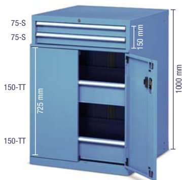
COD. ART. CASSETTI F AE 3040 01 04 4 Armadio con 4 cassetti Dimensioni mm 717x750x1000 h Serratura centrale
