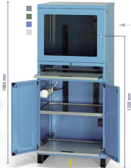
Dim. mm 717x635x1660 h Completo di: 2 piani regolabili in altezza 1 piano porta tastiera 1 piano estraibile 1 coppia zoccoli 100 mm h senza chiusura
