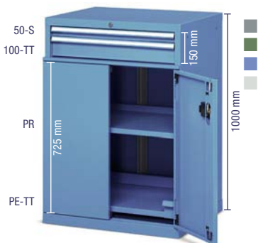
COD. ART. CASSETTI F AE 1040 15 04 2 Armadio con 2 cassetti 1 piano estraibile, 1 piano regolabile Dim. mm 717x597x1000 h Serratura centrale
