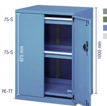
• COD. ART. CASSETTI F AE 2040 01 04 2 Armadio con 2 cassetti 1 piano estraibile Dimensioni mm 717x597x1000 h
