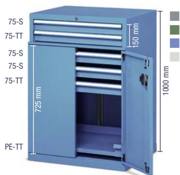
COD. ART. CASSETTI F AE 1040 12 04 5 Armadio con 5 cassetti 1 piano estraibile Dim. mm 717x597x1000 h Serratura centrale
