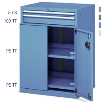
COD. ART. CASSETTI F AE 1040 14 04 2 Armadio con 2 cassetti 2 piani estraibili Dim. mm 717x597x1000 h Serratura centrale
