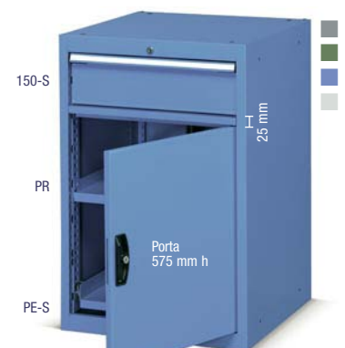
•COD. ART. CASSETTI F DD 1275 51 04 1 Armadio con 1 cassetto ad estrazione semplice 1 piano regolabile, 1 piano estraibile semplice Dim. mm 564x726x850 h Serratura centrale
