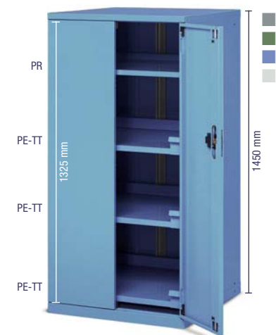
COD. ART. PIANI F AE 4058 10 04 4 Armadio con 3 piani estraibili, 1 piano regolabile Dimensioni mm 717x750x1450 h
