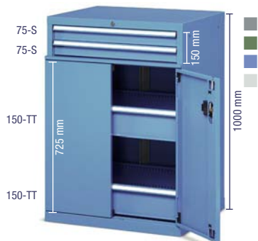
COD. ART. CASSETTI F AE 1040 01 04 4 Armadio con 4 cassetti Dimensioni mm 717x597x1000 h Serratura centrale
