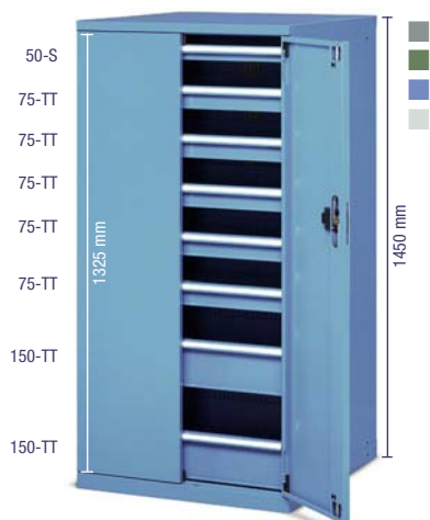
• COD. ART. CASSETTI F AE 4058 12 04 8 Armadio con 8 cassetti Dimensioni mm 717x750x1450 h
