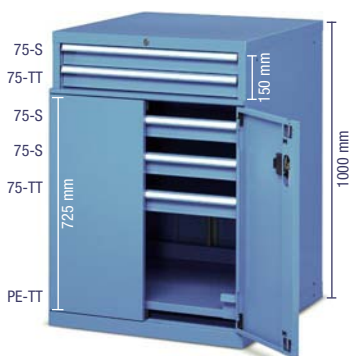
COD. ART. CASSETTI F AE 3040 13 04 5 Armadio con 5 cassetti 1 piano estraibile Dim. mm 717x750x1000 h Serratura centrale
