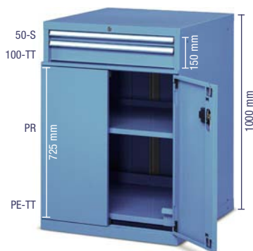
COD. ART. CASSETTI F AE 3040 17 04 2 Armadio con 2 cassetti 1 piano estraibile, 1 piano regolabile Dim. mm 717x750x1000 h Serratura centrale
