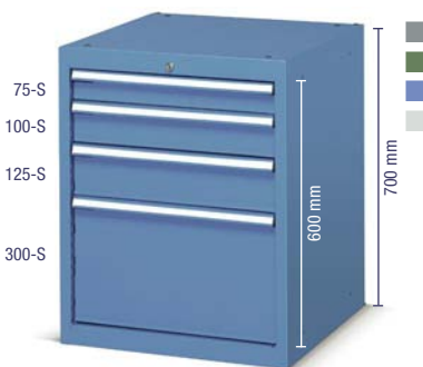
• COD. ART. CASSETTI F DD 1060 54 04 4 Armadio con 4 cassetti ad estrazione semplice Dim. mm 564x726x700 h Serratura centrale
