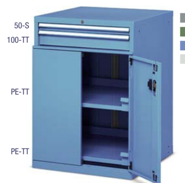
COD. ART. CASSETTI F AE 3040 15 04 2 Armadio con 2 cassetti 2 piani estraibili Dim. mm 717x750x1000 h Serratura centrale
