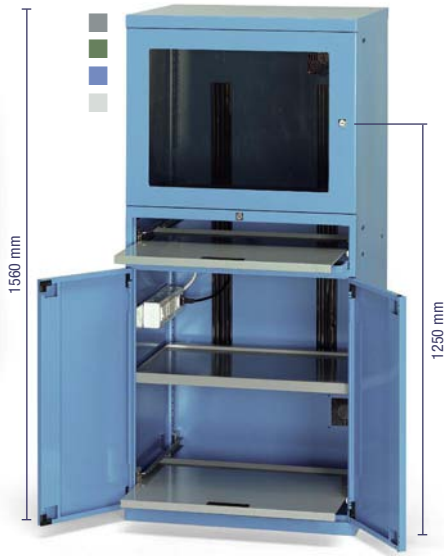
Dim. mm 717x635x1560 h Completo di: 2 piani regolabili in altezza 1 piano porta tastiera 1 piano estraibile
