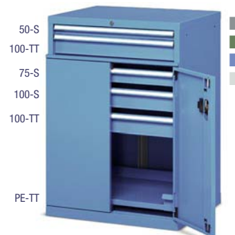
COD. ART. CASSETTI F AE 1040 11 04 5 Armadio con 5 cassetti 1 piano estraibile Dim. mm 717x597x1000 h Serratura centrale
